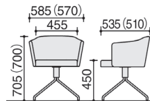
K04-(W.B.M)618·628
