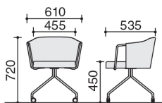
K04-(W·B·M)821
