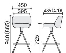
K04-(W·B·M)710·720
