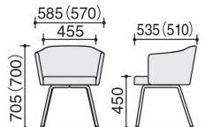
K04-(W·B·M)018·028
