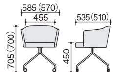
K04-(W·B·M)818·828
