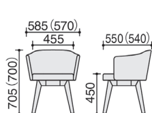
K04-(D·Z)018·028
